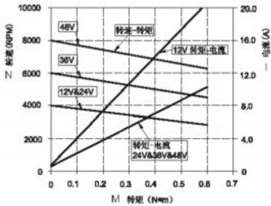
转矩-转速 电流 torque-speed voltage
