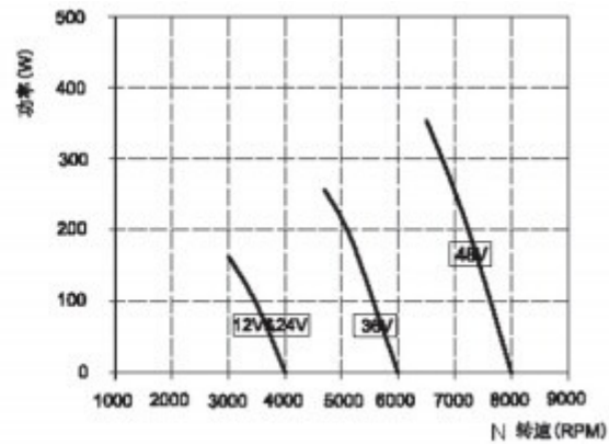
转速-输出功率 speed-output power
